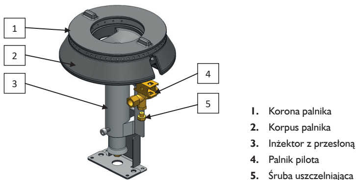
Rysunek 16. Budowa palnika na przykładzie palnika 7kW.
