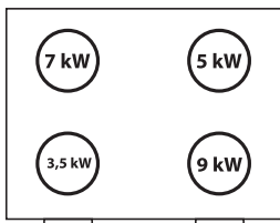
Obrázek 6. Rozmístění hořáků u sporáků se čtyřmi hořáky (schéma)
