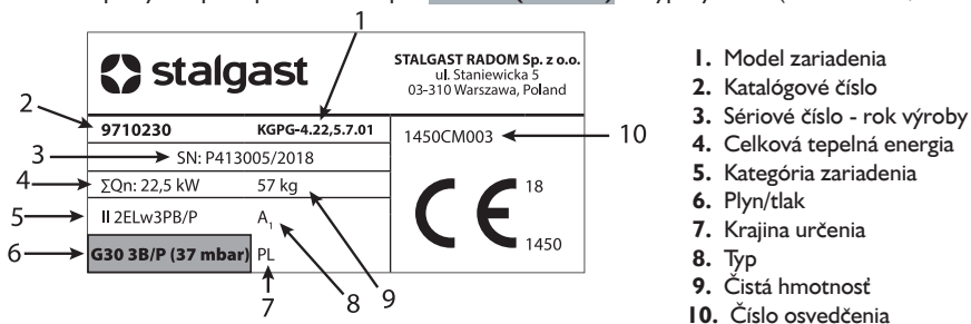
Obrázok 17. Vzor typového štítku
