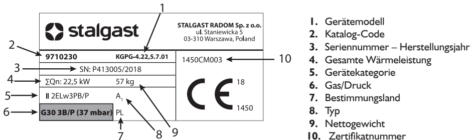
Bild 17. Beispielhaftes Leistungsschild
