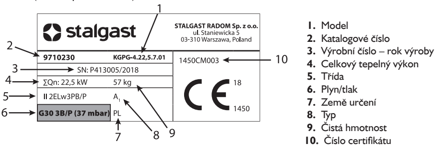
Obrázek 17. Příklad štítku s údaji o zařízení
