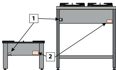
Obrázok 15. Pohľad zo zadnej strany zariadenia.
