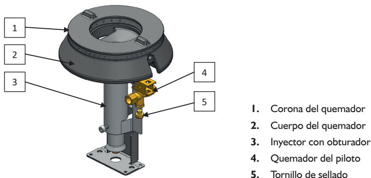
Figura 16. Diseño del quemador sobre el ejemplo de un quemador de 7 kW.
