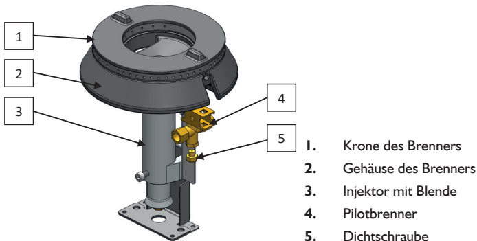
Bild 16. Der Bau des Brenners am Beispiel des Brenners 7kW.
