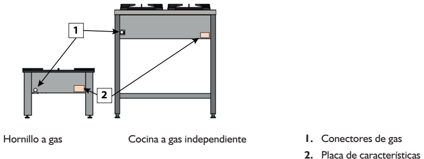
Figura 15. Vista trasera del dispositivo.
