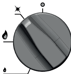
Rysunek 9. Ustawienie pokrętkła w którym zasilany przez gaz jest jedynie palnik pilotowy.
