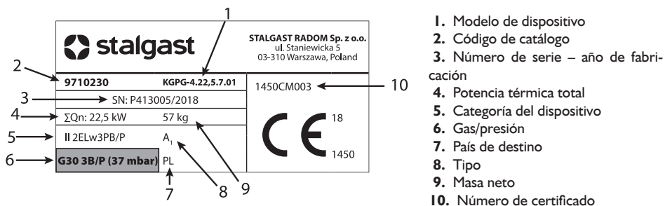
Figura 17. Ejemplo de placa de características
