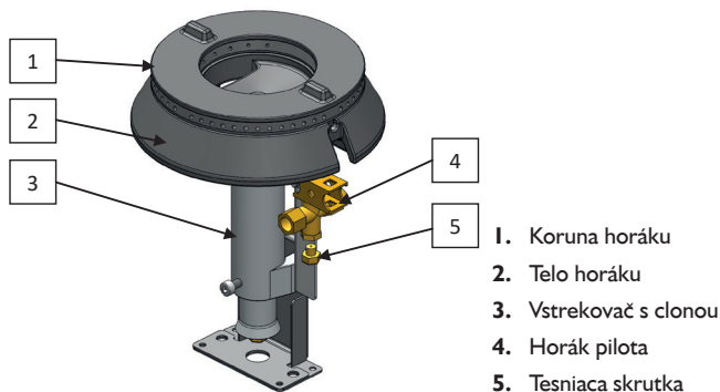
Obrázok 16. Konštrukcia horáku na príklade horáku 7kW.
